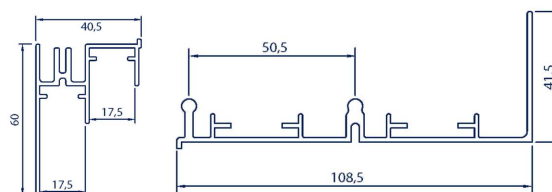
ALU SC01 ajtókhoz, alsó és felső megvezetősín
